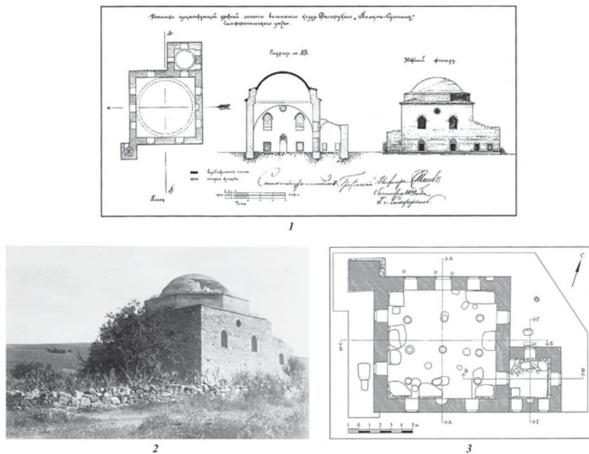
Рис. 7. Мечеть в Пионерском: 1 – чертеж губернского инженера С. П. Иванова 1899 г. «Остатки существующей древней мечети в имени князя Долгорукого «Мамут-Султан» Симферопольского уезда», Картографический фонд библиотеки «Таврика» им. А. Х. Стевена Кру «Центральный музей Тавриды», инв. № 34803 (по В. П. Кирилко, 2012); 2 – старая фотография (автор неизвестен); 3 – план мечети (по В. П. Кирилко, 2012).
