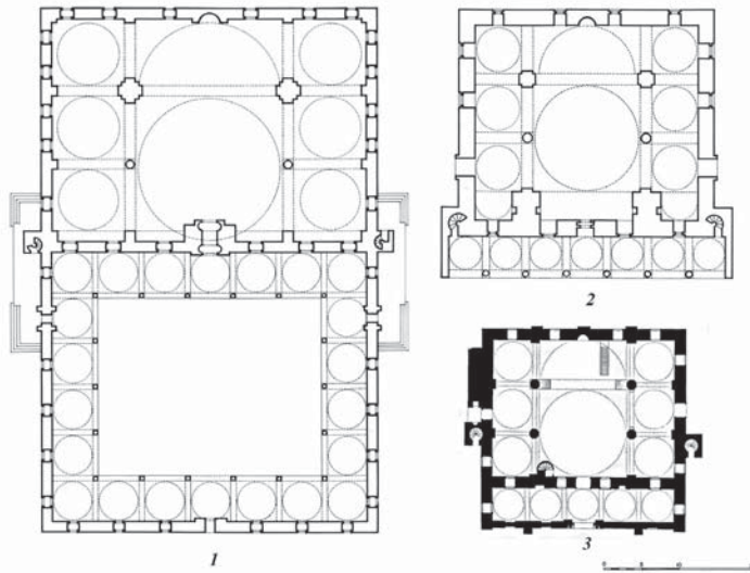
Рис. 25. Османские мечети: 1 – Фатих-джамии в Стамбуле, 1463–71 гг.; 2 – Селимие в Конье, 1566–74 гг. (по Goodwin, 2003); 3 – Джума-Джами в Евпатории, 1552 г.
