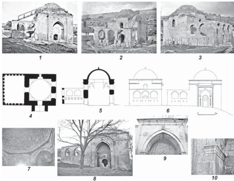
Рис. 48. Эски-Дюрбе в Бахчисарае: 1 – вид с востока; 2 – вид с юга; 3 – вид с запада, фото 1928 г.; 4 – план; 5 – разрез; 6 – южный и восточный; 7 – тропы, фото 1924 г.; 8 – восточный фасад, современный вид; 9 – тимпан арки портала; 10 – карниз пяти арки портала, фасады (по Мирас..., т. 2,3, 2016; фото автора, 2019 г.).
