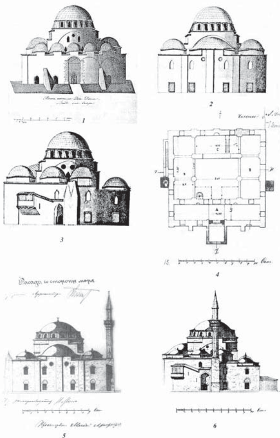
Рис. 22. Джума-Джами в Евпатории: 1 – северный фасад; 2 – южный фасад; 3 – восточный фасад, рис. И. Якубинского, 1836 г.; 4 – план А. Е. Геккера, 1892 г.; 5 – южный фасад; 6 – восточный фасад, рис. А. Е. Геккера, 1892 г. (по В. А. Кутайсов, Кутайсова, 2007).
