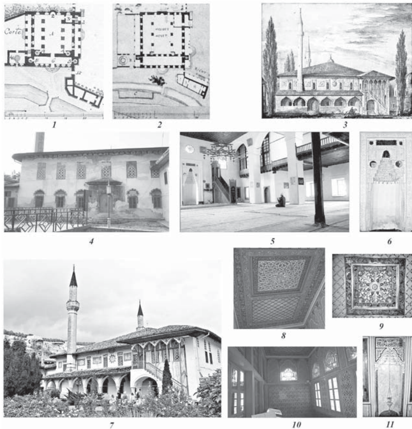
Рис. 27. Большая Ханская мечеть в Бахчисарае: 1 – план, фрагмент плана дворца Джакомо Тромбаро, 1787 г.; 2 – план, фрагмент плана дворца В. Гесте 1798 г.; 3 – вид западного фасада, Кирстен, 1840 г.; 4 – вид северного фасада; 5 – интерьер; 6 – ниша михраба; 7 – вид западного фасада; 8–9 – потолок в ханской ложе; 10 – интерьер ханской ложи; 11 – михраб в ханской ложе (фото автора).
