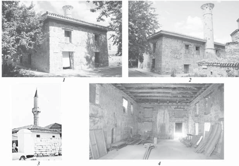
Рис. 33. Мечеть Шукурла-эфенди в Евпатории: 1 – вид с юго-запада; 2 – вид с юго-востока (фото 2019 г.); 3 – минарет до реставрационных работ 1986 г. (по В. А. Кутайсов, Кутайсова, 2007); 4 – интерьер (фото автора, 2019 г.).
