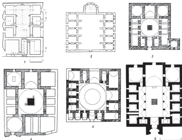
Рис. 43. Текие и медресе Малой Азии: 1 – текие в Баяликёе; 2 – медресе Али Паша в Дьярбакре; 3 – медресе Юсуфа бен Якуба; 4 – Каратай-медресе в Конье; 5 – Чукур-медресе в Токате; 6 – Хатуние в Карамане (по R. Hillenbrand, 1994; Е. И. Кононенко, 2017а).
