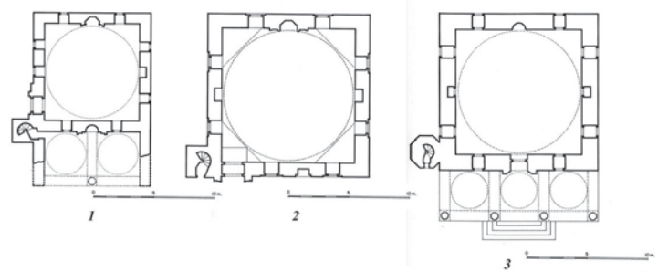
Рис. 16. Купольные мечети Турции османского периода: 1 – Хаси Сахабеддин Паша в Эдирне; 2 – Касим Паша в Эдирне; 3 – Фируз Ага в Стамбуле (по А. Куран, 1971).
