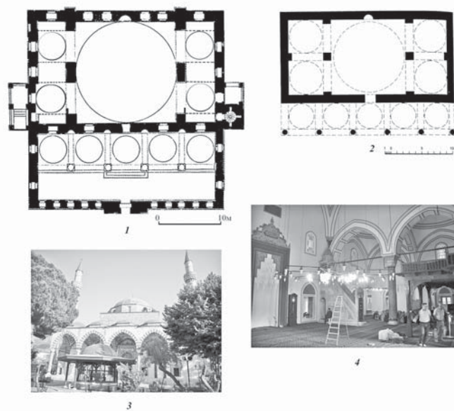
Рис. 20. 1 – мечеть Селима в Феодосии, план с элементами реконструкции; 2 – Султан-Джами в Манисе 1522 г., план; 3 – Султан-Джами в Манисе, северный фасад; 4 – интерьер (фото Е. И. Кононенко).
