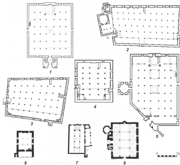
Рис. 34. Турецкие мечети с деревянным плоским перекрытием: 1 – Сахиб-Ата-Джами в Конье, 1279–80 гг.; 2 – Улу-Джами в Афьоне, 1272; 3 – Улу-Джами в Зиврихисаре, 1274–75 гг.; 4 – Ахи-Середеддин-Джами в Анкаре, 1289–90 гг.; 5 – Эшрефоглу-Джами в Бейшехире, 1277 г.; 6 – Махмуд-бей-джами в Касабакее, XIV в.; 7 – Улу-джами в Байбурте, 1283–1298; 8 – Сунгур-бей-Джами в Нигде, 1335 г. (по Hayes, 2010; Кононенко, 2017а).
